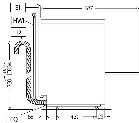
Bočna/o
